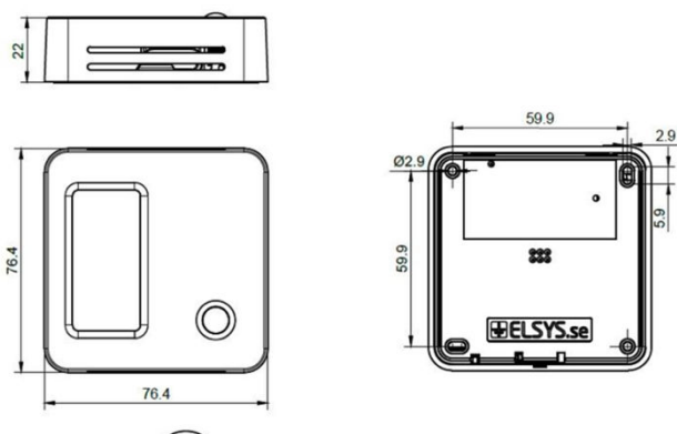
Figur 1. Omni-skärmens mått
